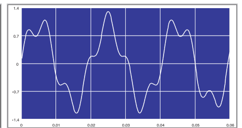
间谐波波形
